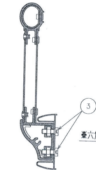
A-A断面図(1/2)
